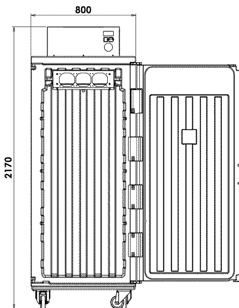
Modello frigo tetto ventilato
